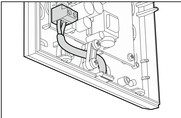
Abb. 2. Befestigung des Kabels zur Stromversorgung.
