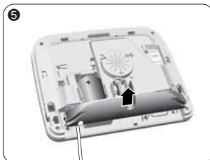
Zdjąć maskownicę gniazda.
