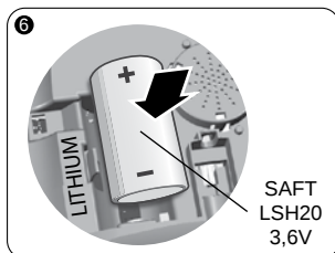
Plaats de batterij, rekening houdend met de polariteit.
