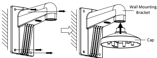
Abbildung 2-13 Montage der Wandhalterung
