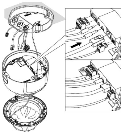
Abbildung 2-9 Kabel verbinden
