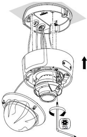
Abbildung 2-10 Befestigen des Kameragehäuses
