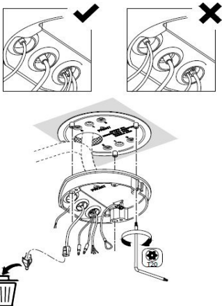
Abbildung 2-7 Kabel durch die Anschlussdose verlegen
