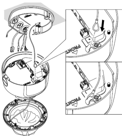
Abbildung 2-8 Anschlussdose montieren
