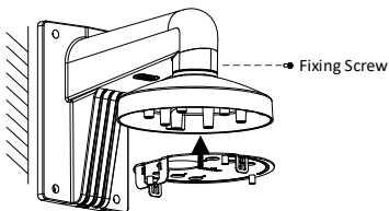
Abbildung 2-14 Montage der Adapterplatte an der Kappe
