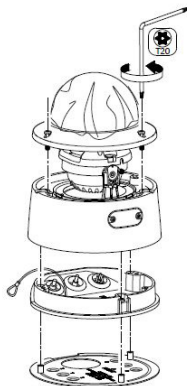
Abbildung 2-2 Demontage der Kamera
