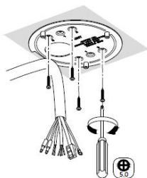
Abbildung 2-3 Adapterplatte
