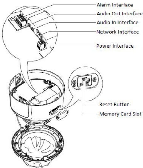
Abbildung 1-1 Überblick über die Dome-Kamera
