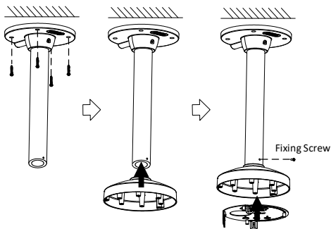
Abbildung 2-15 Abgehangene Halterung montieren
