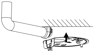
Abbildung 2-5 Rohrleitung montieren
