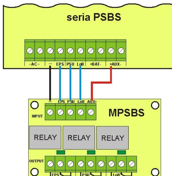
Abb. 5. Anschlussschema des MPSBS-Moduls.
