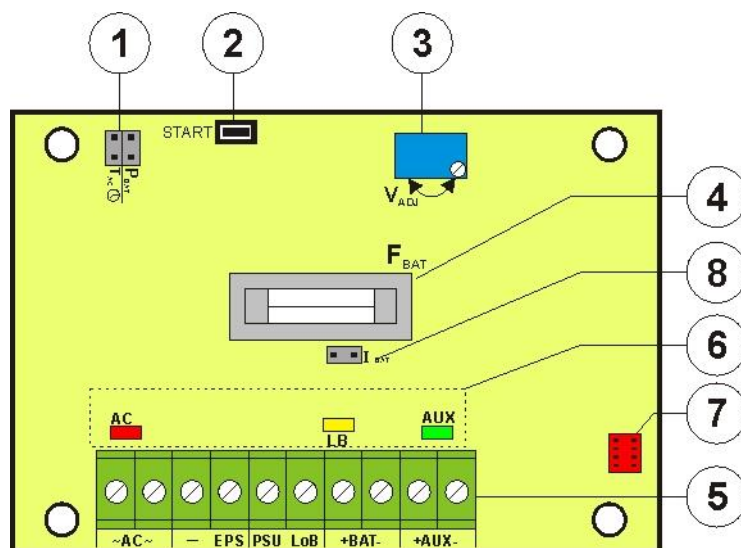
Abb. 2. Ansicht PCB-Platte des Netzteils.
