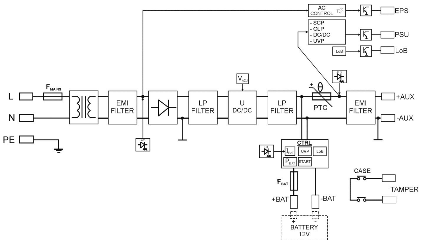
Abb. 1. Blockschaftbild des Netzteils.
