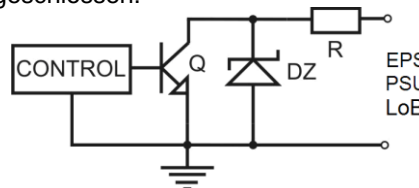
Abb. 4. Elektroschaltbild des OC-Ausgänge.
