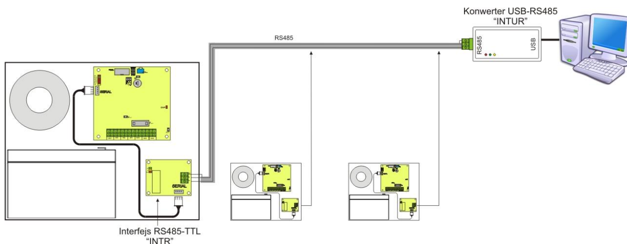
Abb. 30. Kommunikation RS485 mit der Nutzung des Interfaces „INTR“ und „INTUR“.
