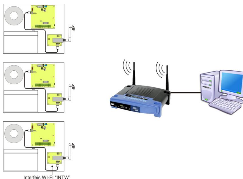
Abb. 28. Kommunikation Wi-Fi mit der Nutzung des Interfaces Wi-Fi „INTW“.
