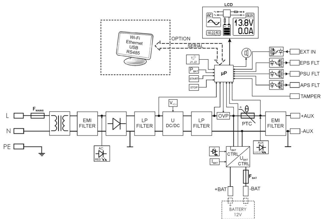
Abb. 1. Das Blockschemata des Netzgeräts.
