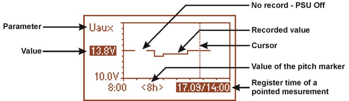
Abb. 12. Bildschirm der Geschichte der Parameter des Netzgeräts.
