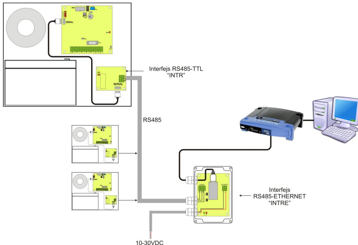
Abb. 27. Kommunikation Ethernet mit der Nutzung des Interfaces RS485-Ethernet „INTRE“.
