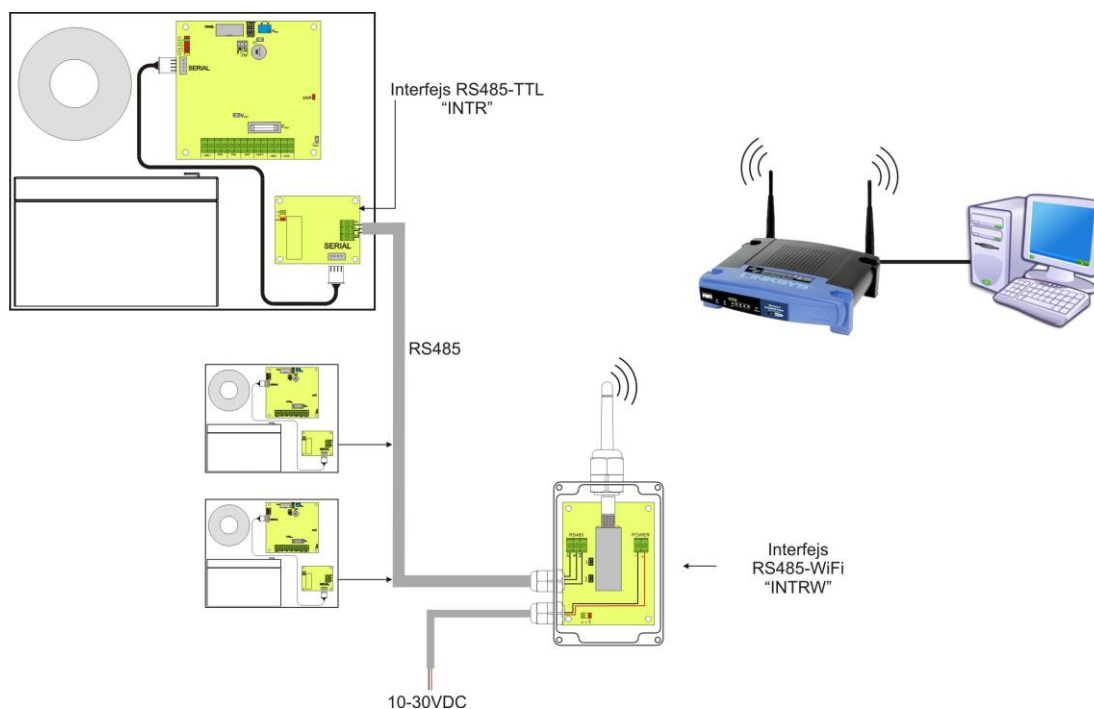
Abb. 29. Kommunikation Wi-Fi mit der Nutzung des Interfaces RS485-WiFi „INTRW“.
