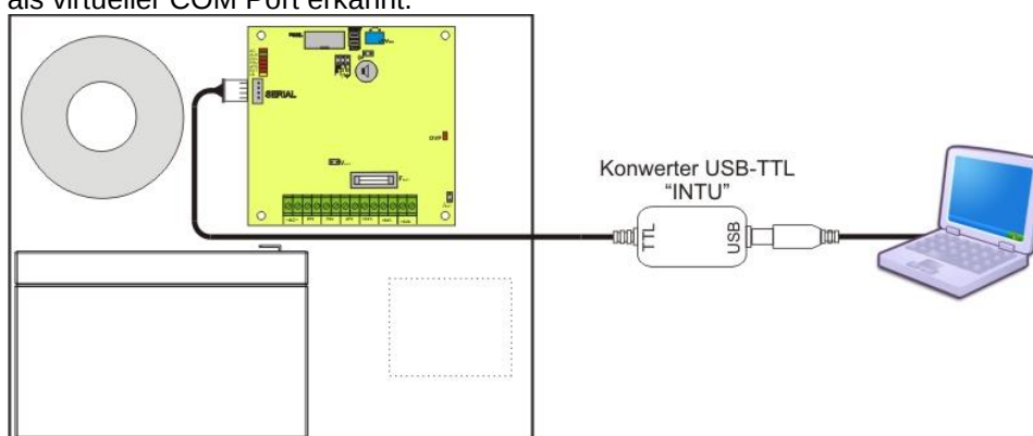
Abb. 25. Kommunikation USB-TTL mit der Nutzung des Interfaces USB-TTL „INTU“.
