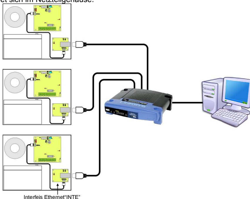
Abb. 26. Kommunikation Ethernet mit der Nutzung des Interfaces Ethernet „INTE“.
