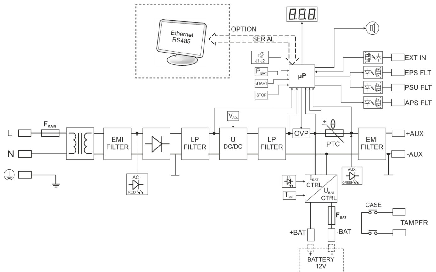
Abb. 1. Das Blockschemata des Netzgeräts.
