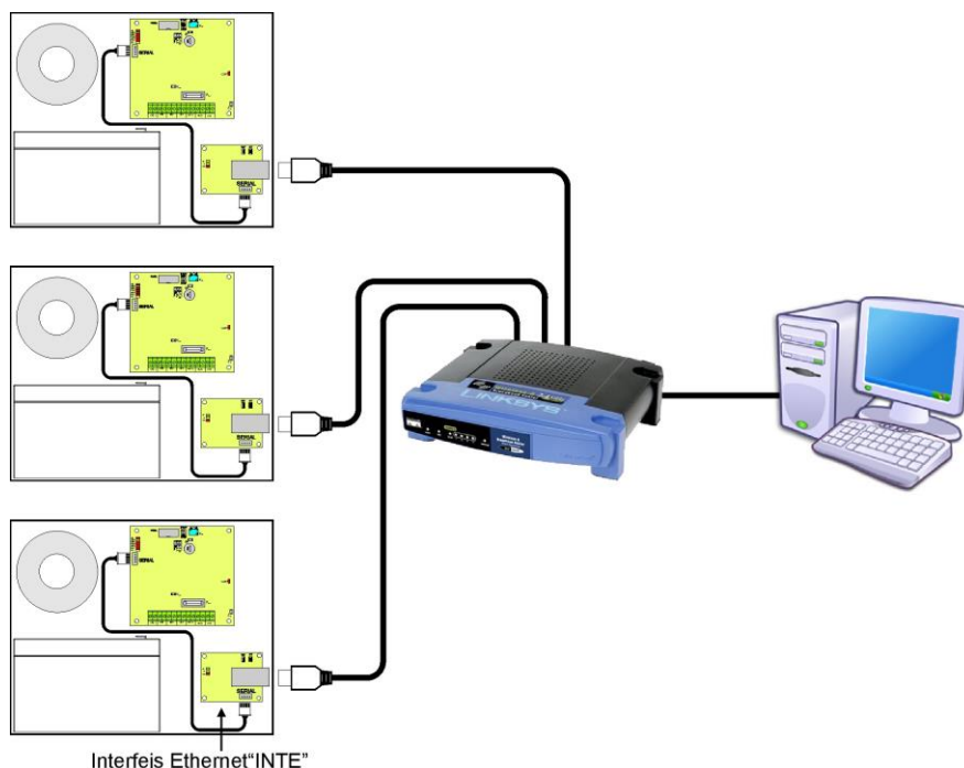
Abb. 12. Kommunikation Ethernet mit der Nutzung des Interfaces Ethernet „INTE“.
