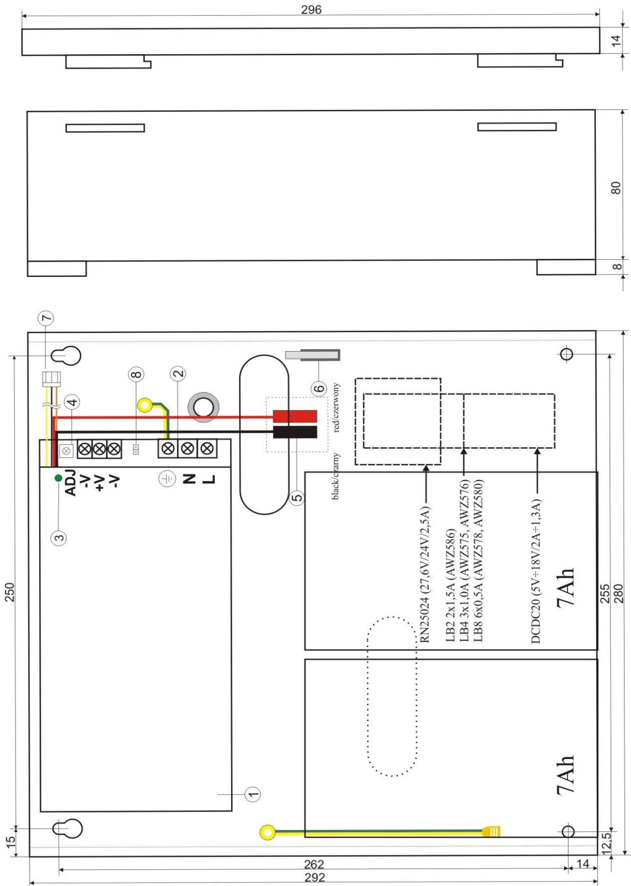
Bild 2. Netzteil-Ansicht.
