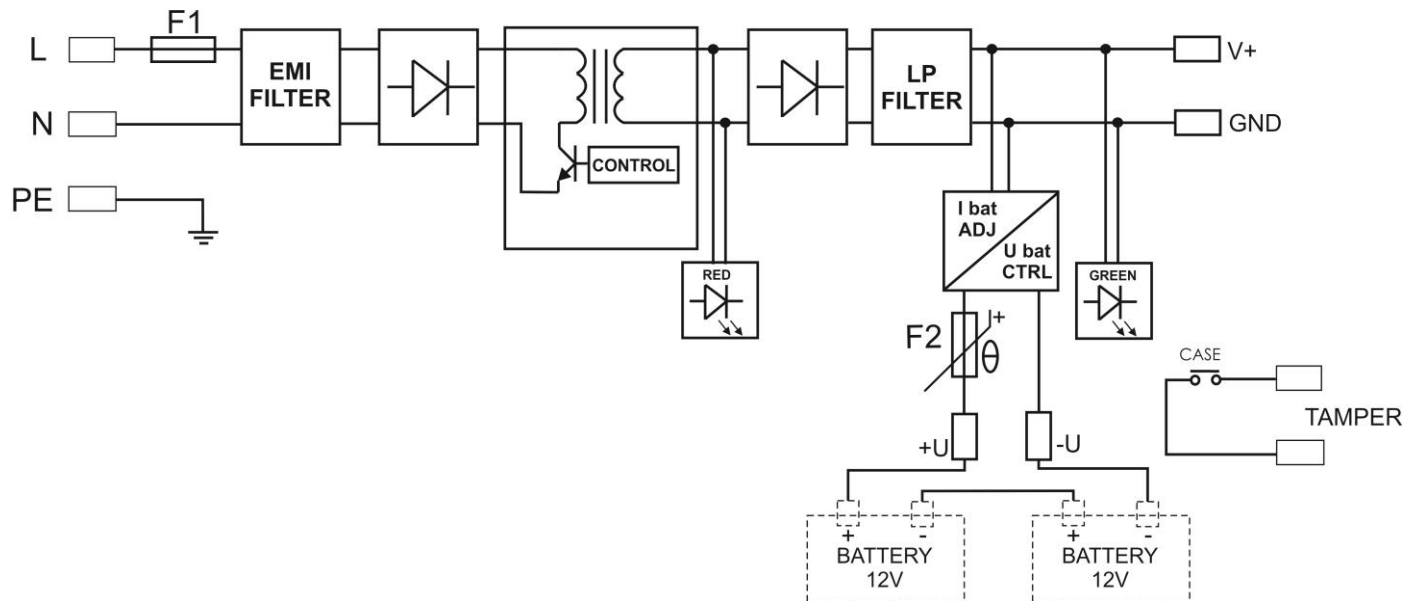
Bild 1. Schaltplan Netzteil.
