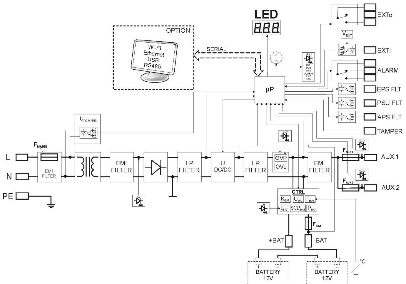
Abb. 1. Das Blockscheema des Netzgeräts.
