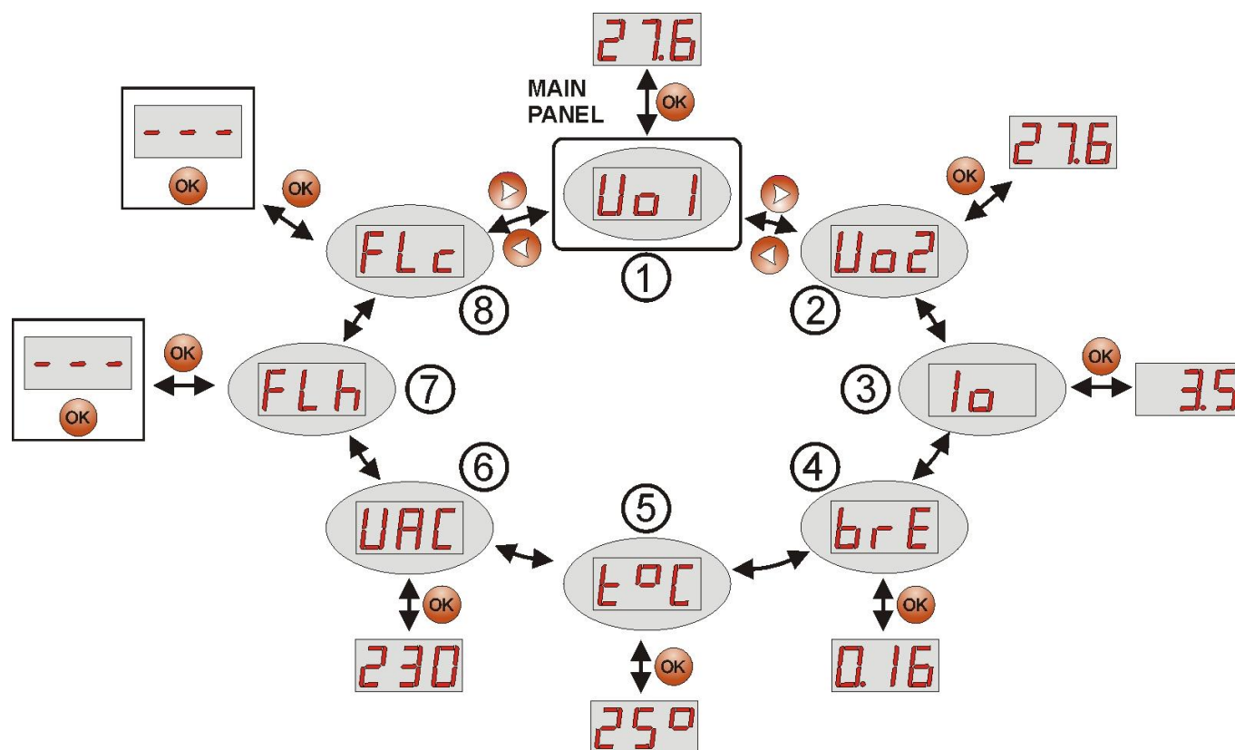
Abb. 8. Menü des Netzgeräts.
