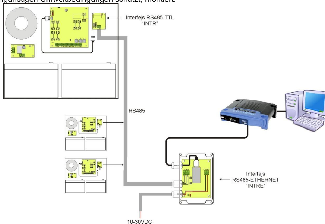
Abb. 17. Die Ethernet – Kommunikation unter Verwendung des RS485-Ethernet „INTRE“-Interfaces.
