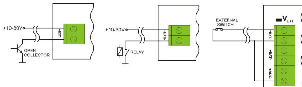
Abb. 12. Beispielhafte Anschlussweisen.
