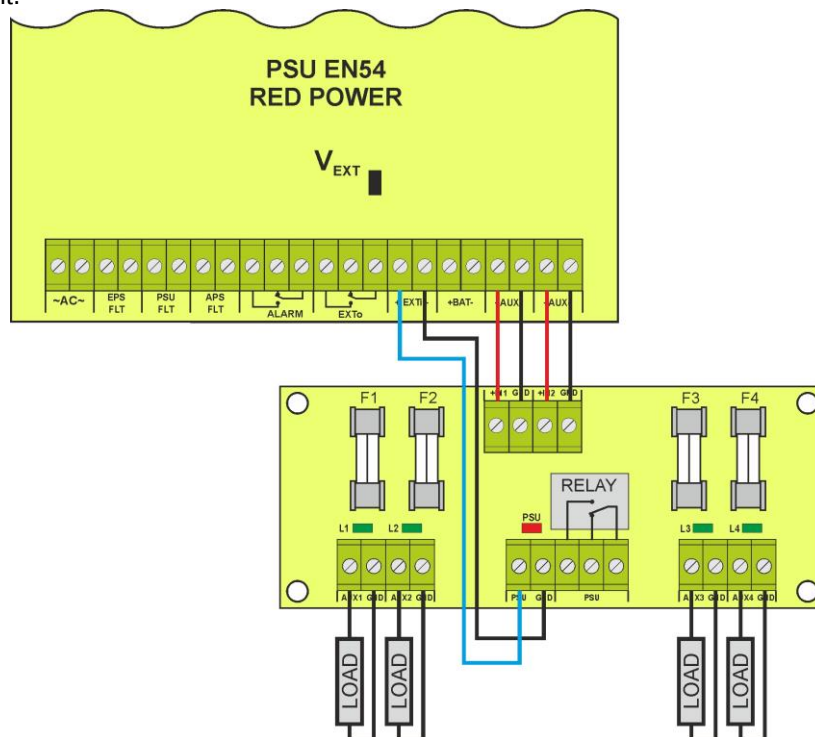
Abb.14. Anschlussweise des Sicherungsmoduls.
