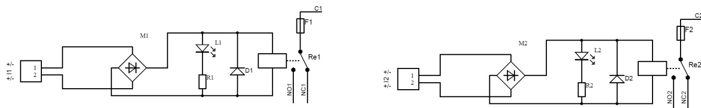
Abb. 2. Elektrisches Schema.
