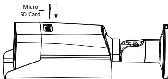
Abbildung 2-2 Speicherkarte einsetzen
