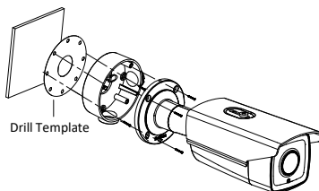
Abbildung 2-7 Montage mit Anschlussdose
