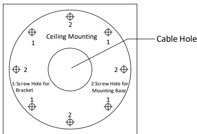
Abbildung 2-2 Bohrschablone
