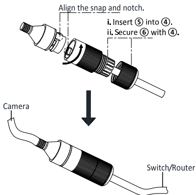
Abbildung 2-10 Installation der wasserdichten Schutzhülle
