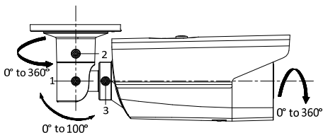
Abbildung 2-4 Anpassen des Blickwinkels
