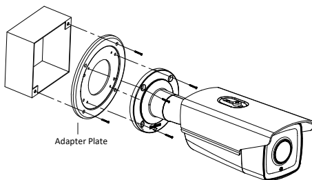
Abbildung 2-8 Montage mit einer Unterputzdose
