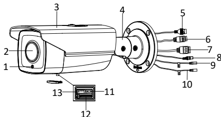
Abbildung 1-1 Kamera Übersicht
