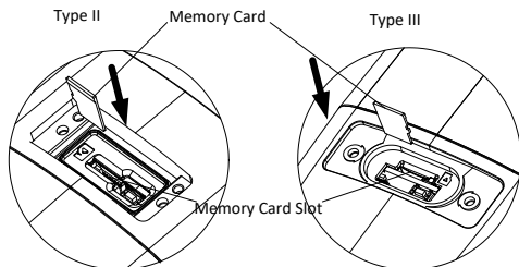
Abbildung 2-2 Speicherkarte einsetzen
