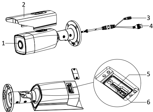
Abbildung 1-1 Bullet Kamera Überblick
