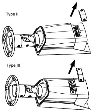
Abbildung 2-1 Speicherkartensteckplatz freilegen
