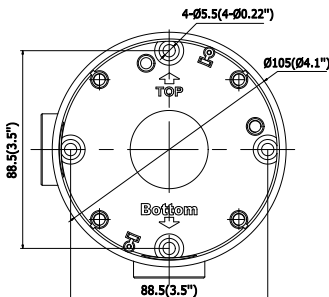
Abbildung 2-6 Abmessungen der Anschlussdose
