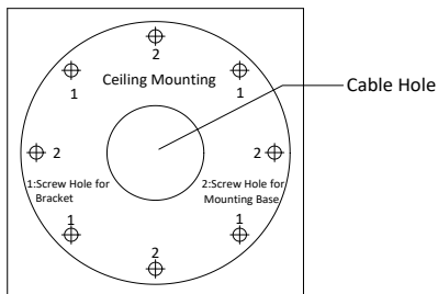
Abbildung 2-2 Bohrschablone
