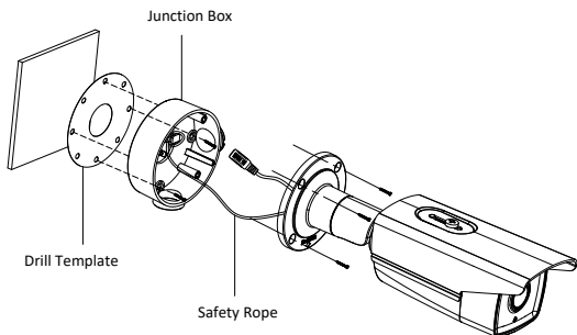
Abbildung 2-7 Montage mit einer Anschlussdose
